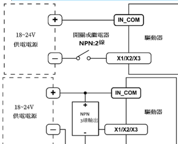
輸入迴路
