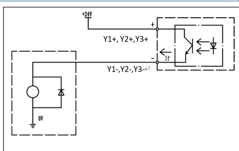
輸出迴路
